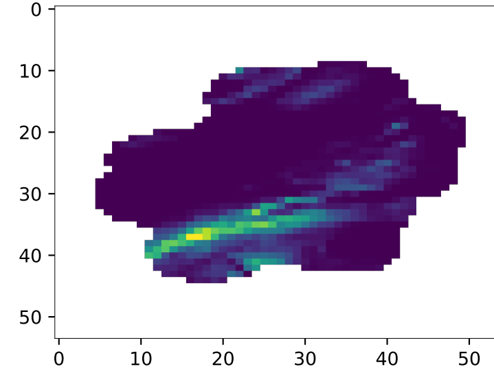
target (RADKLIM)
