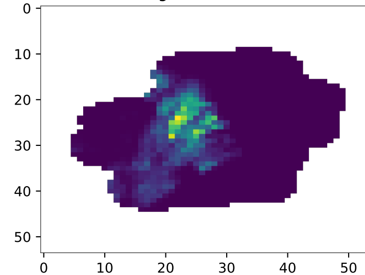
target (RADKLIM)
