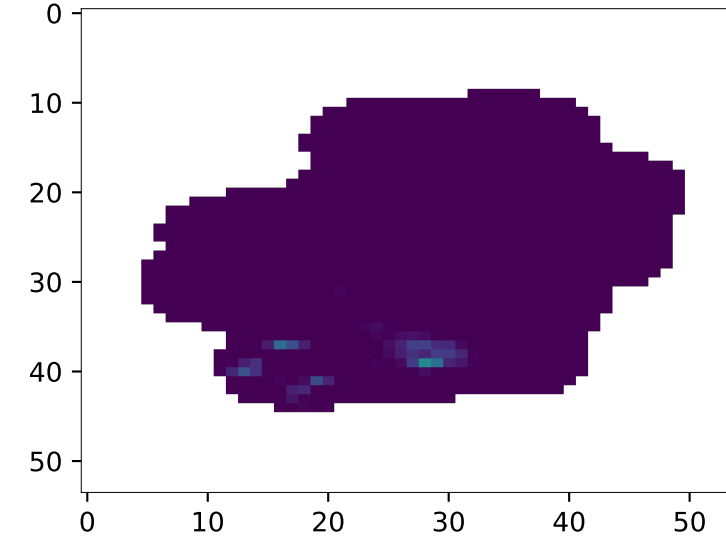
target (RADKLIM)
